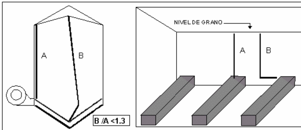
Figura II: Relación entre distancias menores y mayores de recorrido del aire en una celda.
